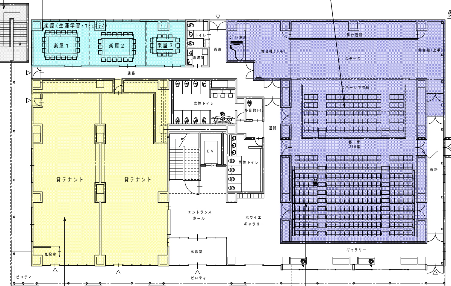
1 階 平 面 図
